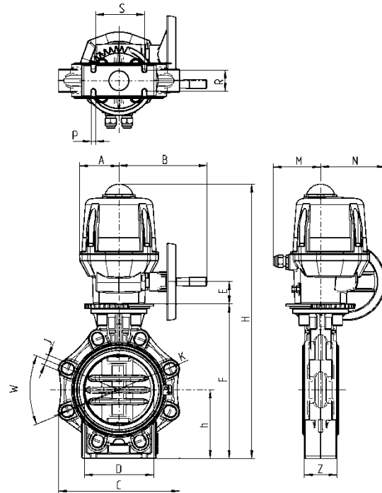
Actuator VS150 / VS300
